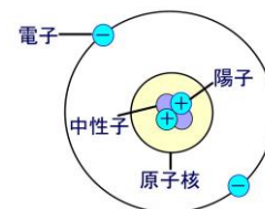
ヘリウム原子の構造
