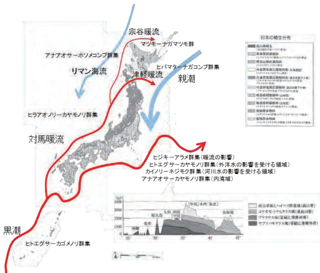
図 3-1 日本を取り巻く海流と植生（陸生植生と海藻植生）
